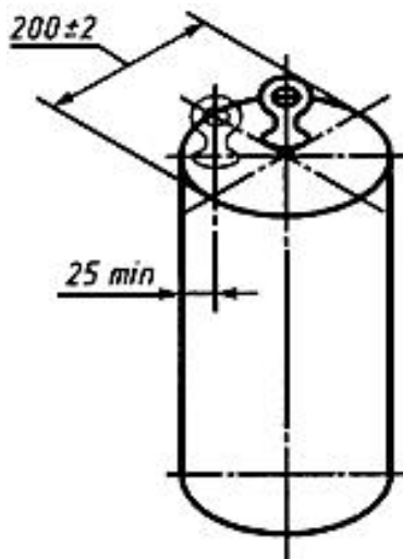
Рисунок 2 - Жесткие стальные грузы (варианты расположения болта)
